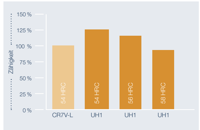
Zähigkeit im Vergleich
