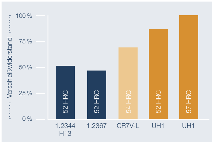
Verschleißwiderstand im Vergleich
