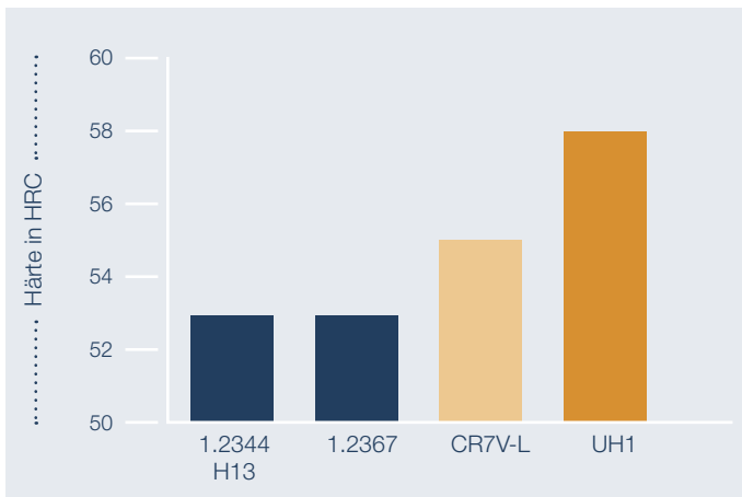
Maximal empfohlene Einsatzhärte
